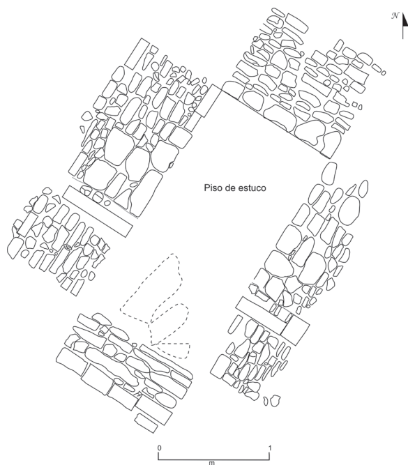
Figura 17. Tumba 13; planta de la tumba con alzados de sus paredes. Dibujo: Felicita López Franco.
