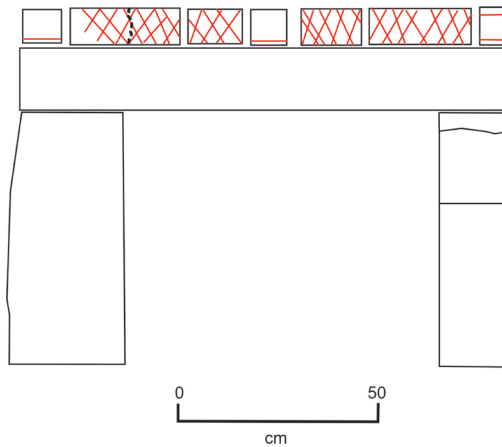
Figura 16. Tumba 13; reconstrucción de la fachada con el dintel y cornisa decorada con piedras de agua y calizas alternadas, ambas pintadas. Dibujo: Felicitas López Franco.
